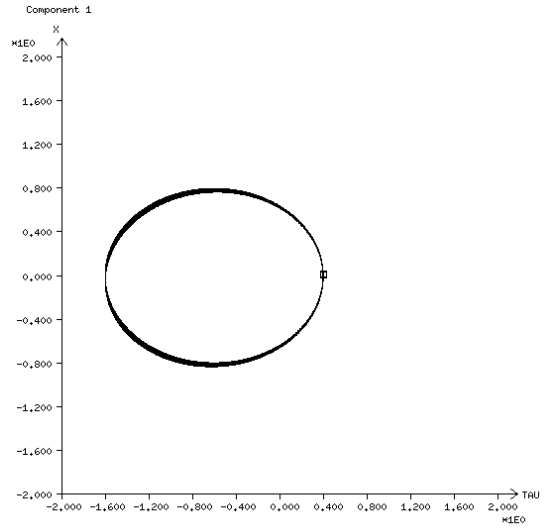
Implizite Mittelpunktsregel auf Mannigfaltigkeit bzgl. H
