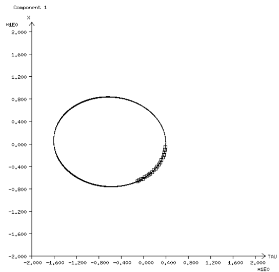
Symplektisches Euler-Verfahren 2
