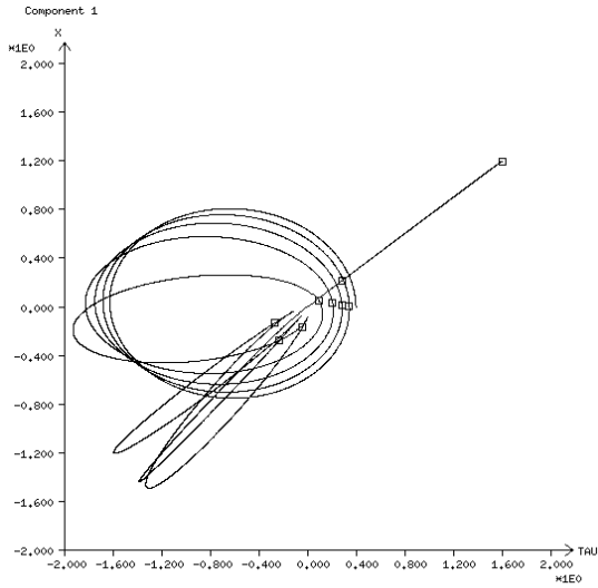
Implizites Euler-Verfahren auf Mannigfaltigkeit bzgl. H
