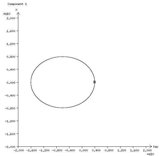
Implizite Mittelpunktsregel auf Mannigfaltigkeit bzgl. H, M, A
