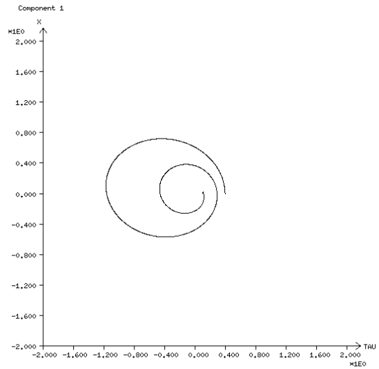
Implizites Euler-Verfahren
