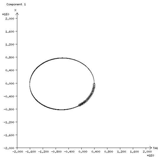
Symplektisches Euler-Verfahren 1
