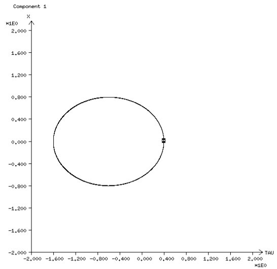
Implizite Mittelpunktsregel auf Mannigfaltigkeit bzgl. H, M
