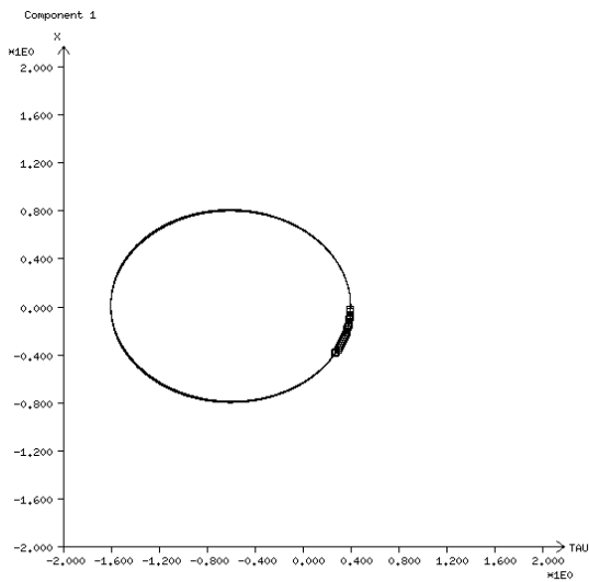
Störmer/Verlet-Verfahren
