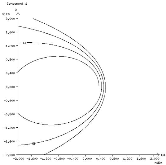
Explizites Euler-Verfahren
