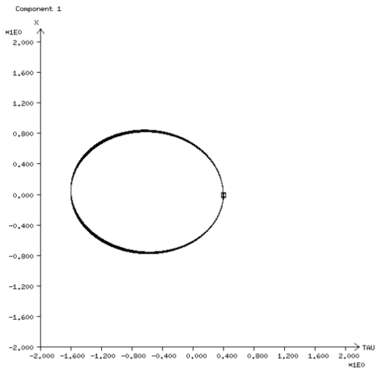
Implizites Euler-Verfahren auf Mannigfaltigkeit bzgl. H, M
